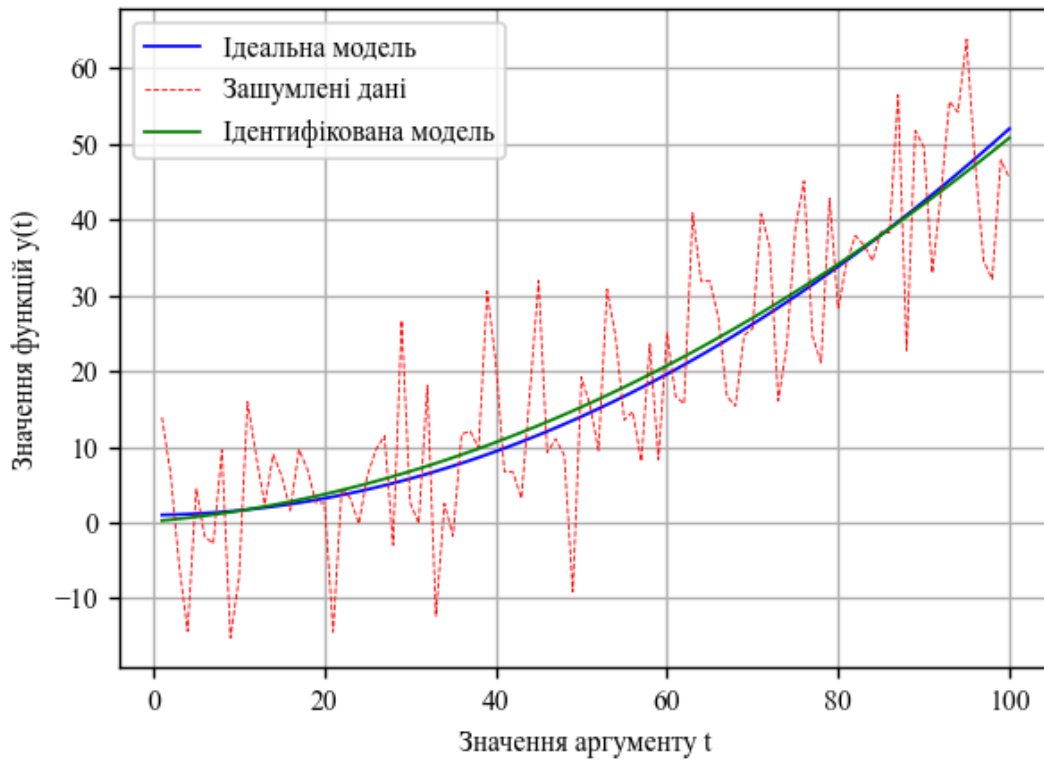
Рисунок 2.2 – Результати параметричної ідентифікації при \text{noise\_level} = 0,5
