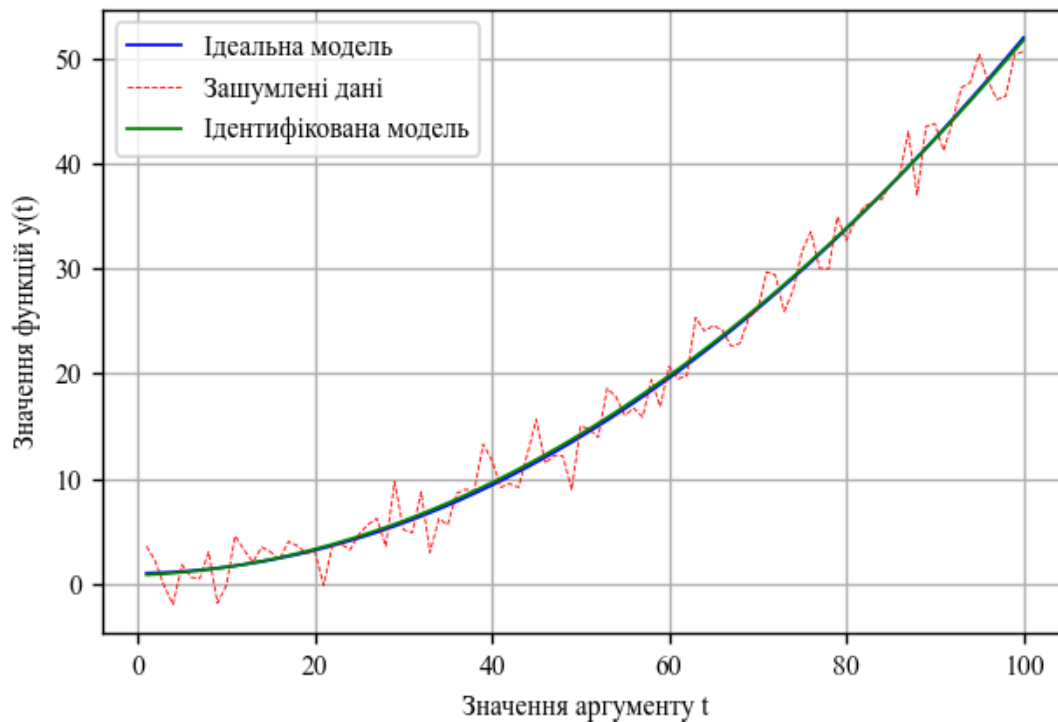
Рисунок 2.1 – Результати параметричної ідентифікації при \text{noise\_level} = 0,1
